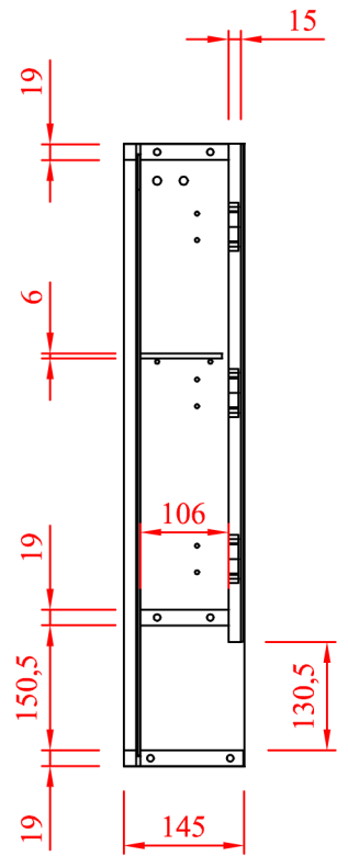
PERFIL
