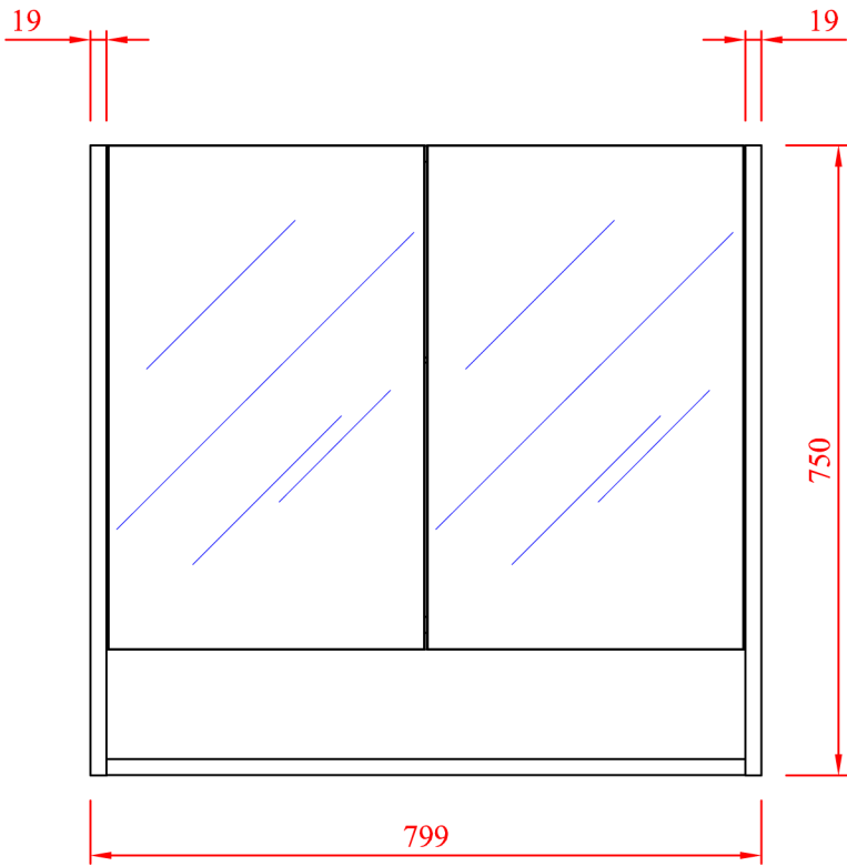
ALZADO
