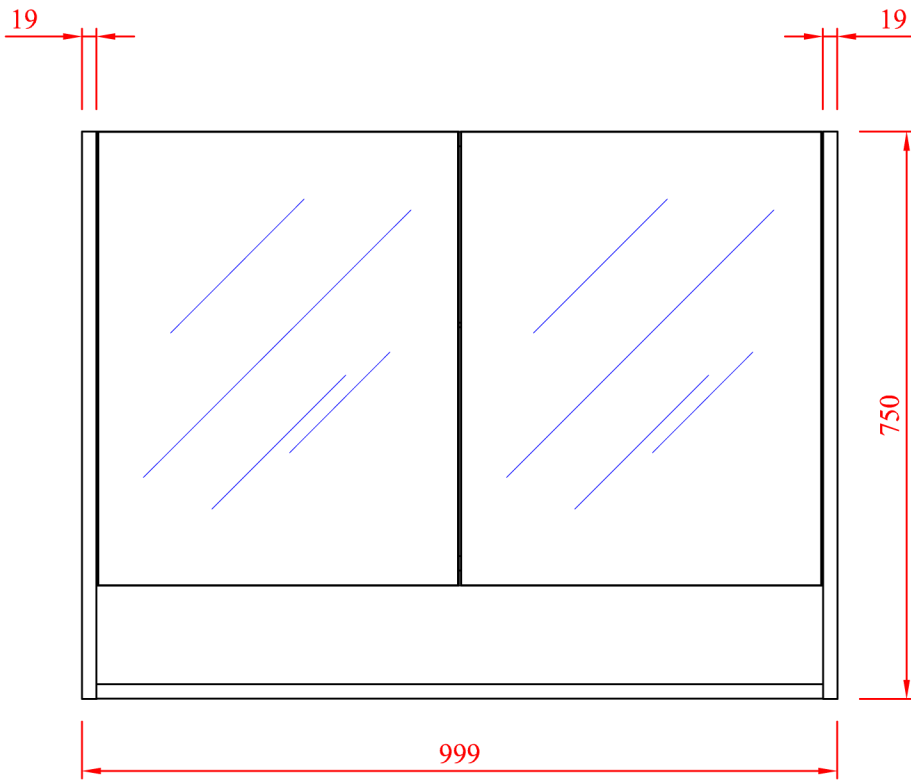
ALZADO
