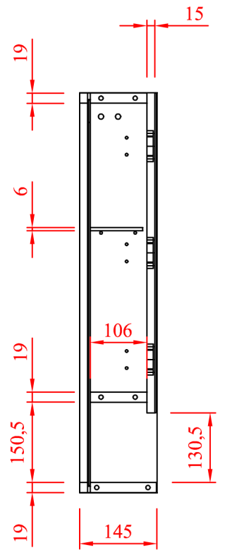
PERFIL
